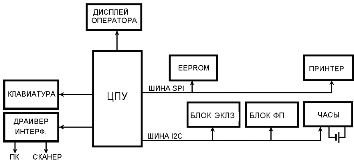
Рис.4. Структурная схема ККМ.
